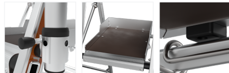
Sistema de despliegue de la barandilla
