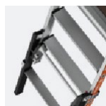
Stufen 80 mm (fester Leiterabschnitt) und 60 mm (teleskopischer Leiterabschnitt)
