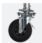
Roues Ø 200 mm à blocage réglables sur 175 mm et tous les 12,5 mm
