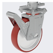
Ruedas de Ø200 mm con bloqueo muy potente y ajuste milimétrico.
