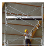
Facilité d'installation des garde-corps monoblocs
