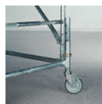
Pieds à roue réglables sur 200 mm tous les 25 mm
