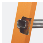
Montants en acier époxy et échelons sertis
