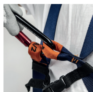
Brustverankerung bestehend aus 2 Gurtschnallen
