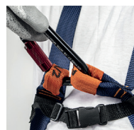
Brustverankerung bestehend aus 2 Gurtschnallen
